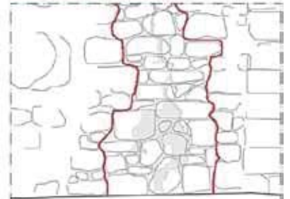
Risarcitura della lesione
