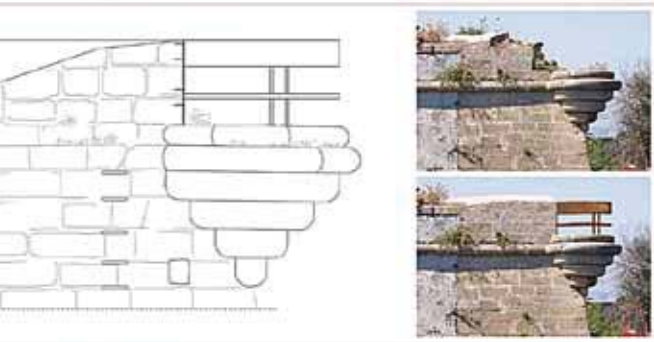
Consolidamento del cantonale
