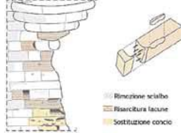
Consolidamento del cantonale
