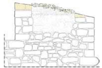
Consolidamento della cresta muraria
